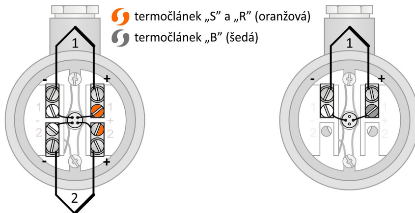
Obrázek 1C.4: zapojení dvojitého termočlánu
